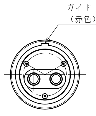
矢視 A - A
